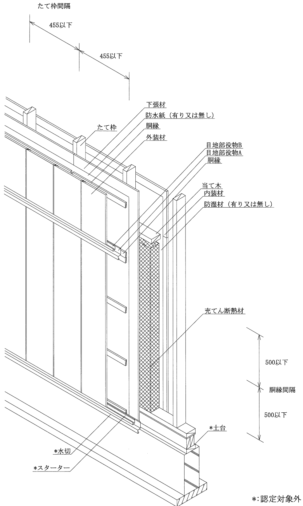
透視図
